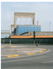
46 PIER LUIGI NERVI: Papierfabrik, Mantua, 1960–64
